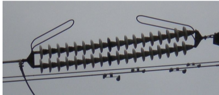
Funkenstrecke bei selbststrahlenden Sendemasten (von (Japanische Zeichen nicht darstellbar) ↗ © ⓘ)
